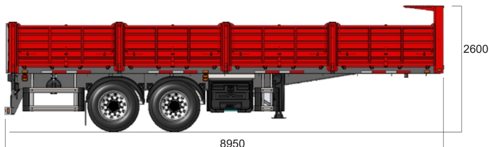
VAGÓN TRASERO: PESO APROX.: 4950 KG
